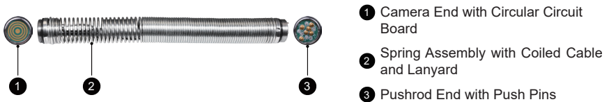
MX Mini Termination Spring Assembly
