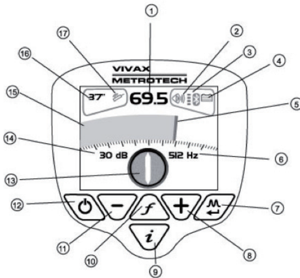
vLocCam2 Receiver Display
